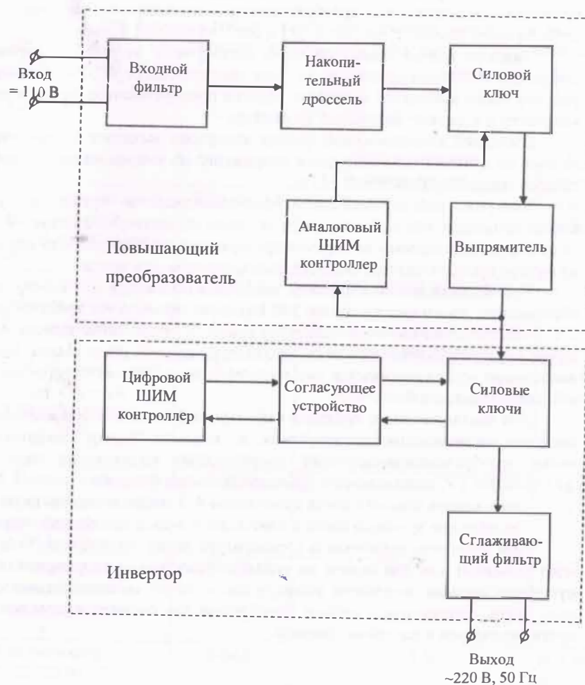
Рисунок 1 - Структурная схема преобразователя
